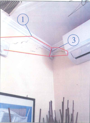
LESIONI N. 1 E N. 3 CORRISPONDENTI ALL'INTERNO DEL LOCALE
