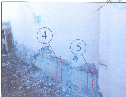
LESIONI N. 4 E 5 SUL CORDOLO DI FONDAZIONE
