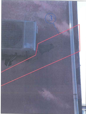
3) LESIONE STRUTTURALE POSTA SUL LATO DESTRO DEL FABBRICATO
