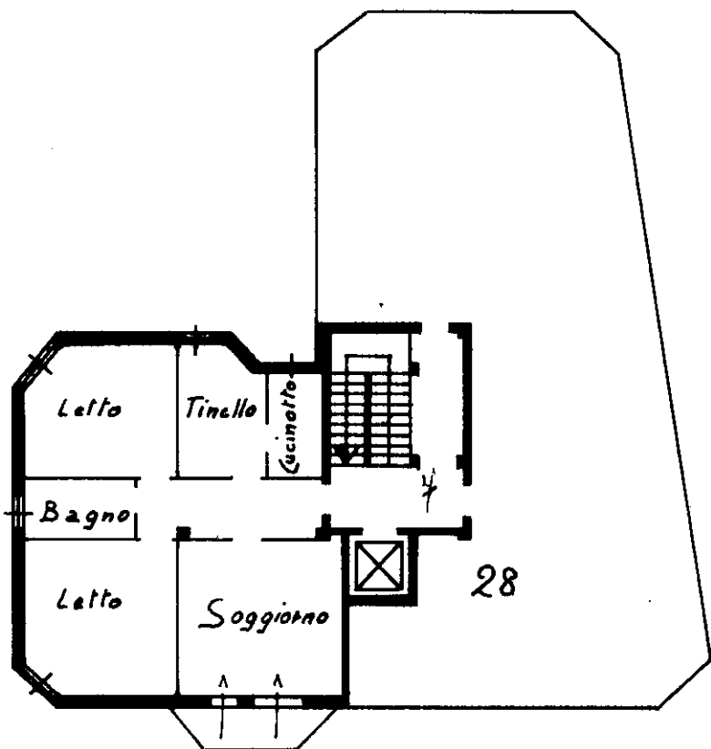
PIANTA TERZO PIANO h: 2.80
