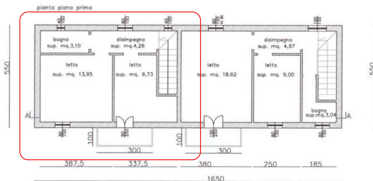
Schema spazi piano primo – parte fabbricato a Sx come da riquadro rosso
