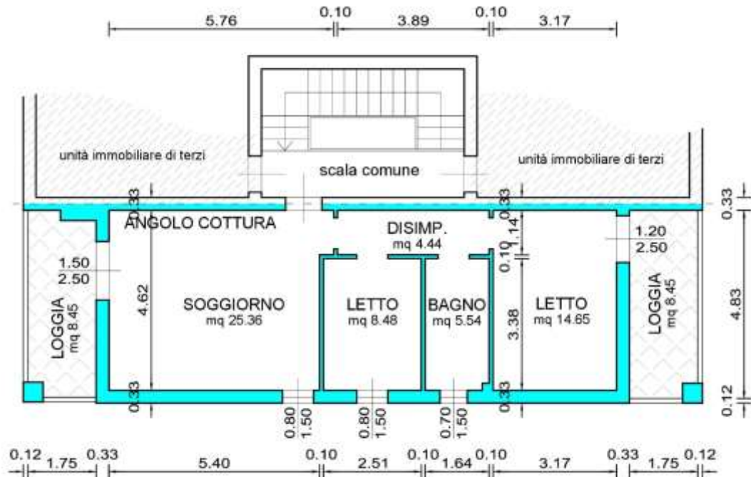
PIANTA PIANO SECONDO H 270
