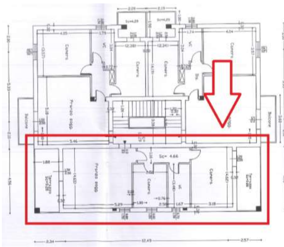
PIANTA PIANO SECONDO H 270
