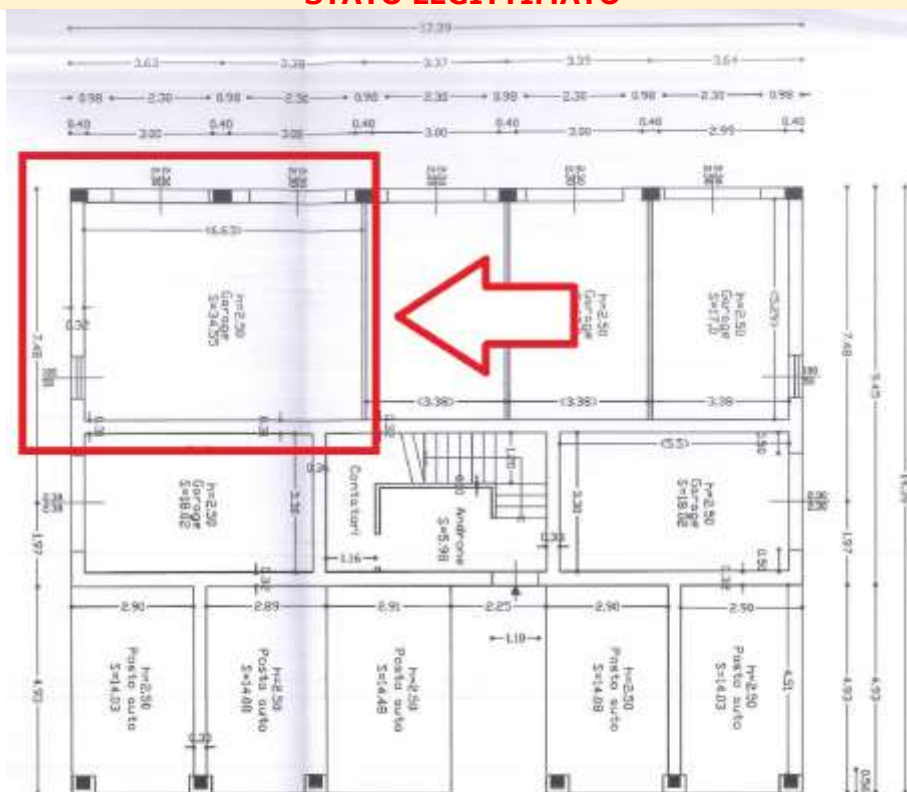
PIANTA PIANO TERRA H 250
