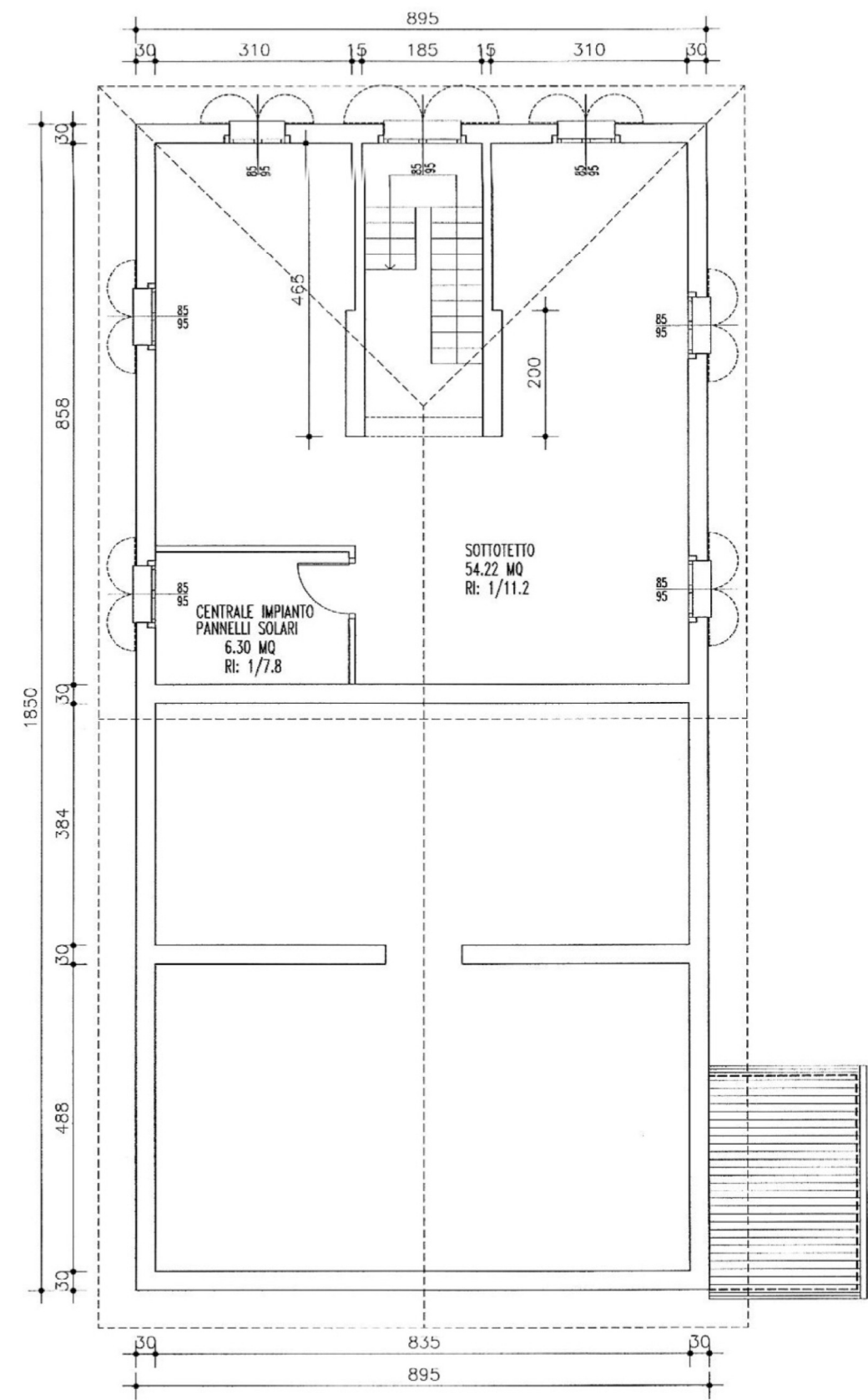
PIANO SOTTOTETTO
