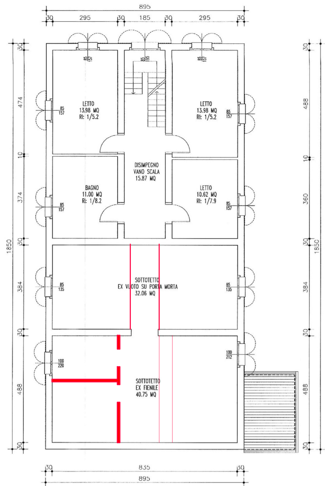
PIANO PRIMO
