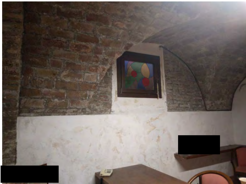
Foto n. 11 – uno scorcio del grande vano centrale posto nel seminterrato, ben visibili le volte di laterizio in foglio e le vaste zone ammalorate a causa dell'umidità di risalita e contro-terra
