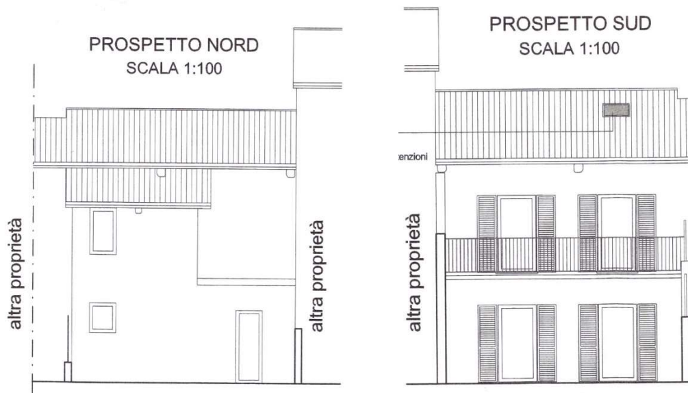
Fig. 9 - Le rappresentazioni dell'edificio viste da nord e da sud allegata alla DIA del 2005
