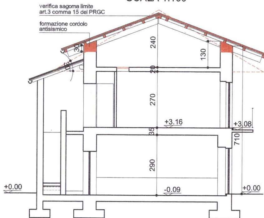
Fig. 10 – Le sezioni dell'edificio allegate alla DIA del 2005
