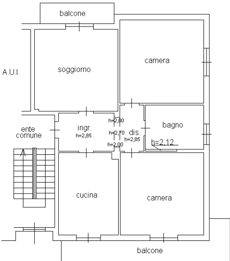
PIANO SECONDO h=3,05
