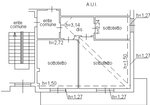
PIANO TERZO (sottotetto)
