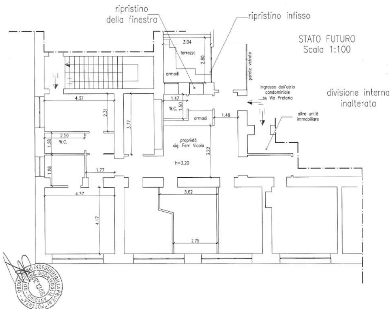
Figura 6 - Pianta piano terra allegata alla "D.I.A. Denuncia di Inizio Attività" prot. n. 1061 del 8.1.2010"
