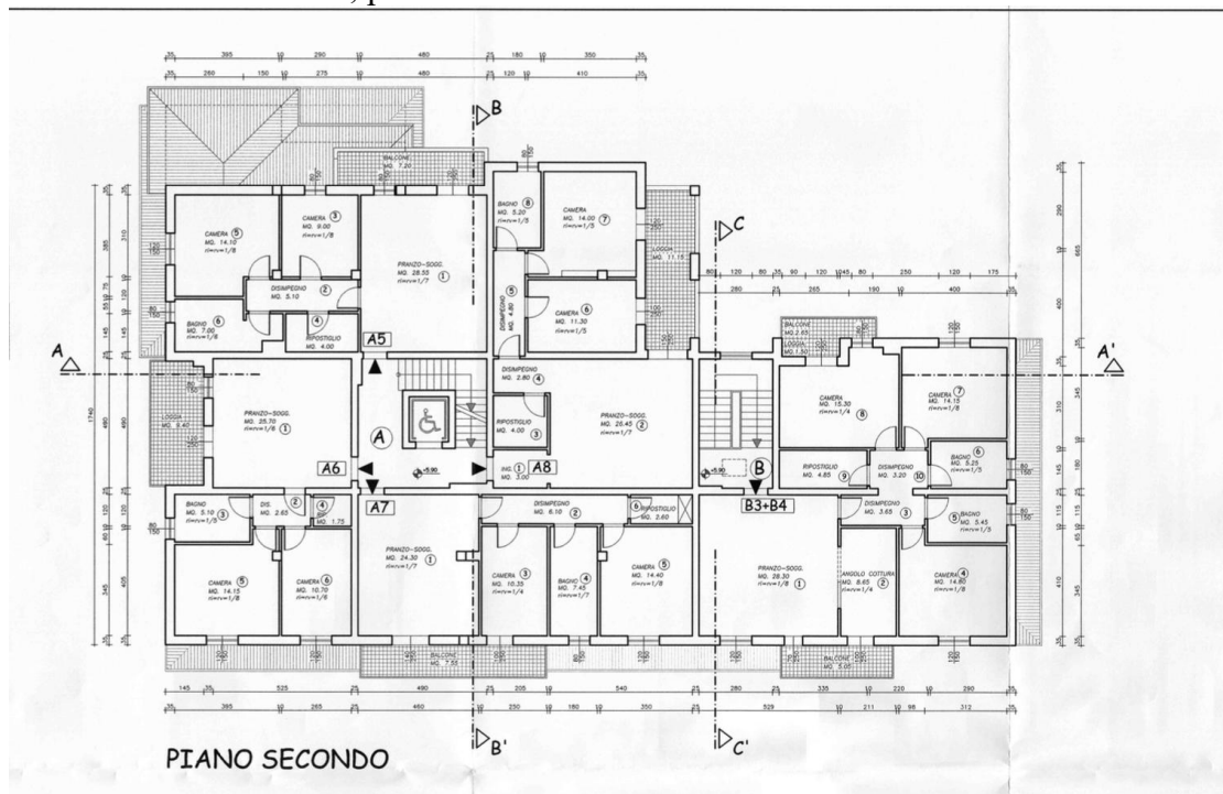
Ultimo stato autorizzato, secondo piano
