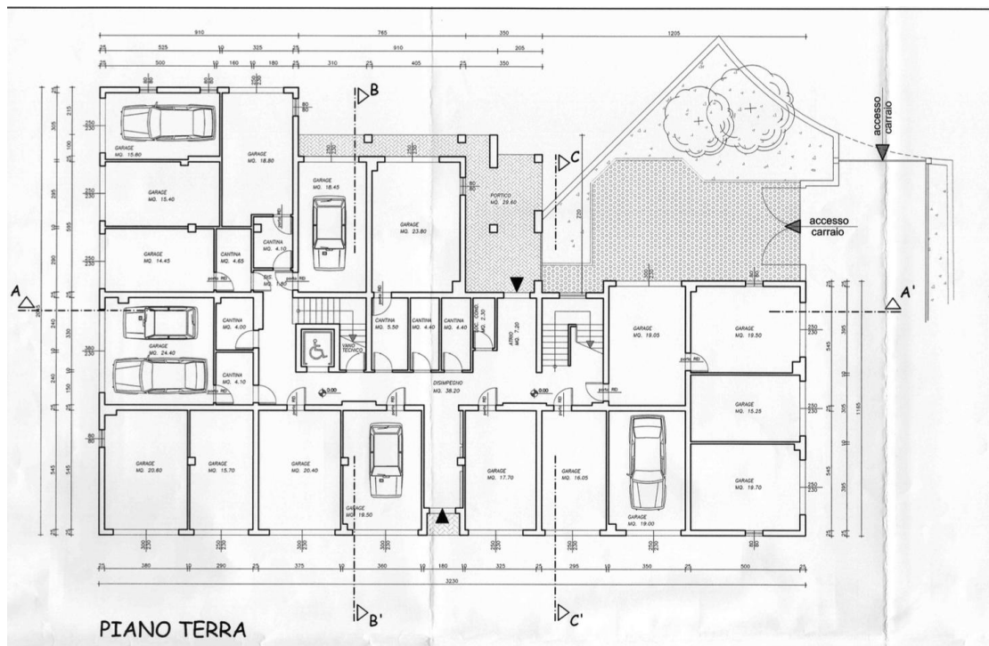
Ultimo stato autorizzato, piano terra
