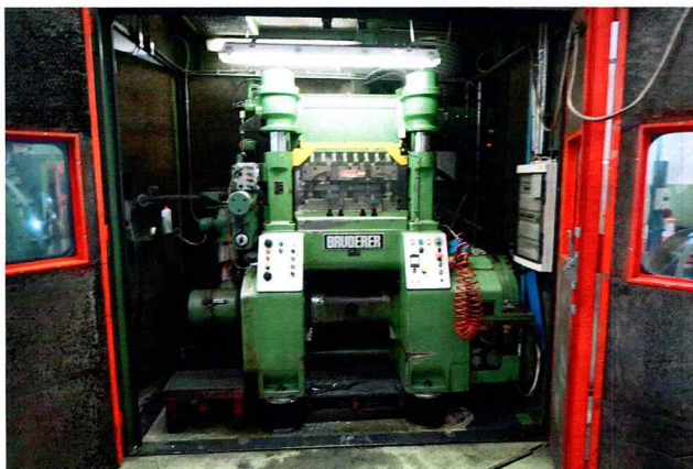
Foto 13 – T04 – Pressa Bruderer BSTA 60L – matricola 3134
