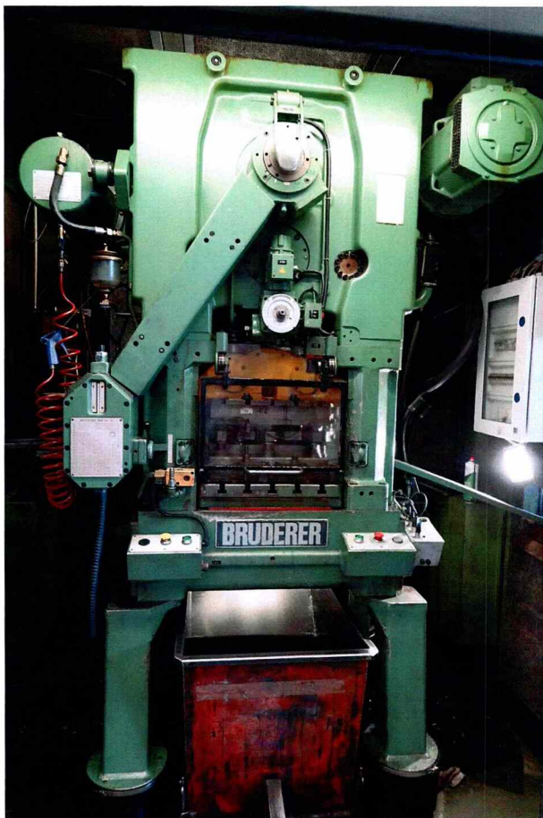
Foto 10 – T03 – Pressa Bruderer BSTA 25H – matricola 9807
