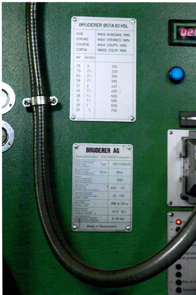
Foto 17 – T05 – Pressa Bruderer BSTA 60HSL – matricola 9644
