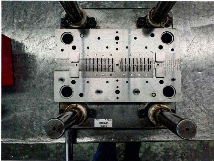
Foto 38 – Ref. 003 Tool da 17mm a 31mm 1P
