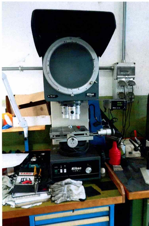
Foto 26 - Rif. 143 - PROIETTORE PROFILI NIKON
