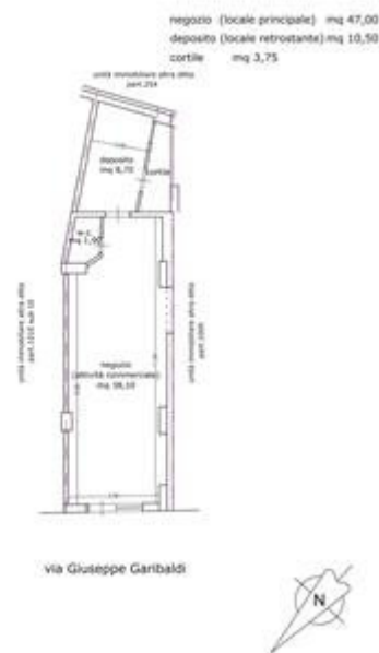
rilievo planimetrico stato di fatto
