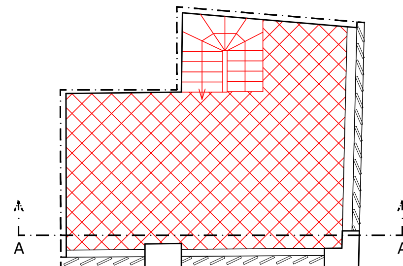
PIANO SECONDO
