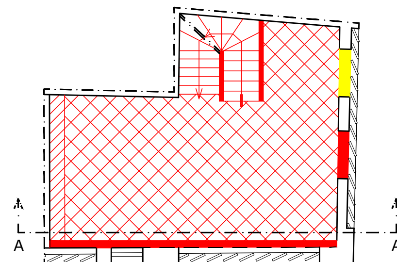
PIANO PRIMO
