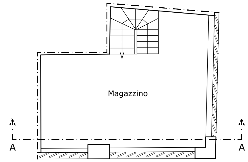
PIANO SECONDO
