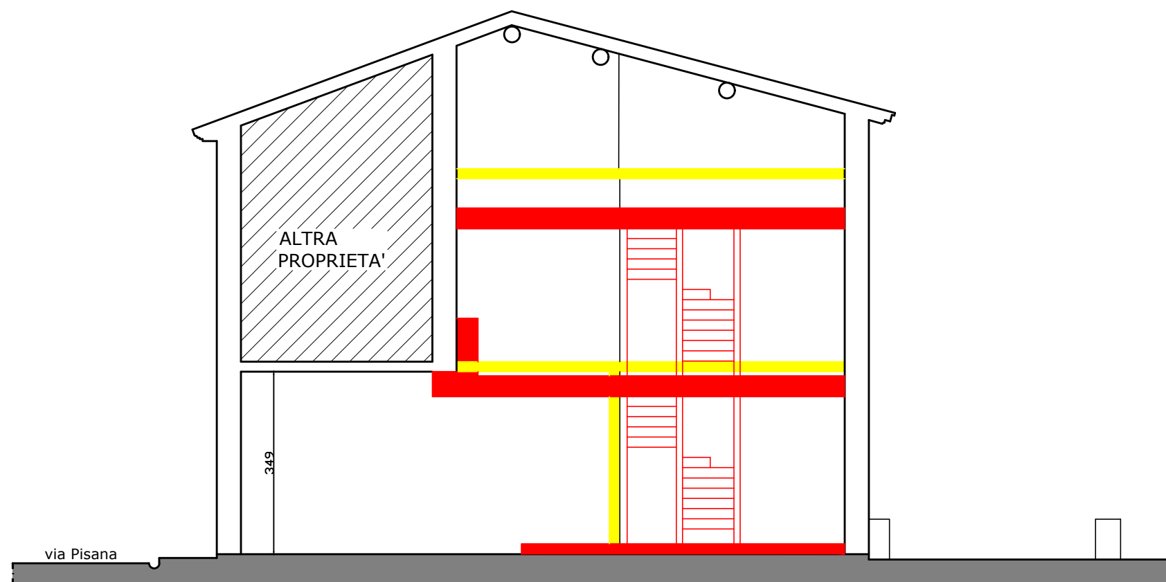
SEZIONE A-A
