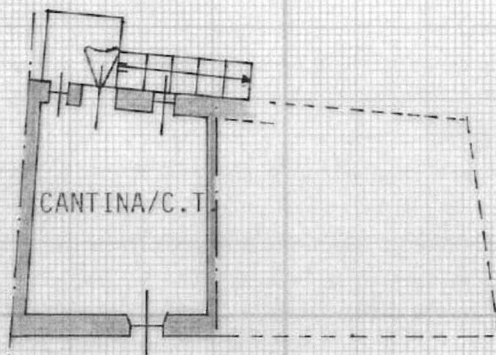
PIANTA PIANO INTERRATO H. media 2.20
