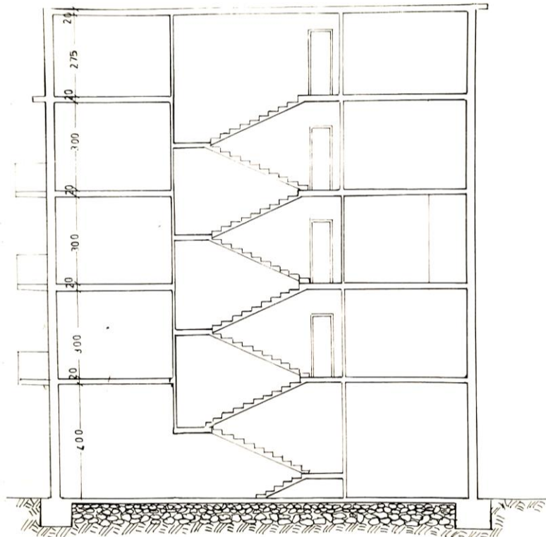
SEZIONE A-A'
