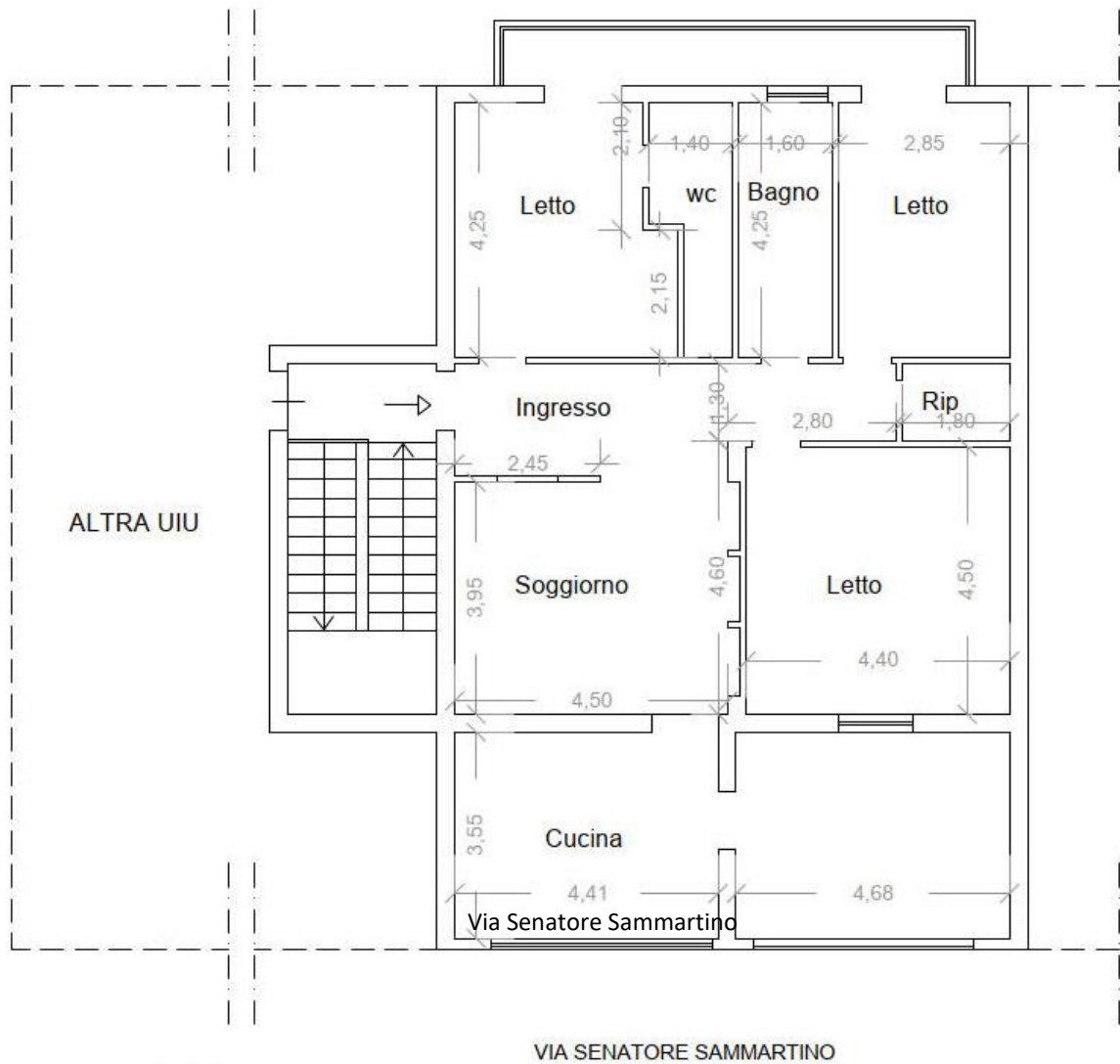
Planimetria quotata
