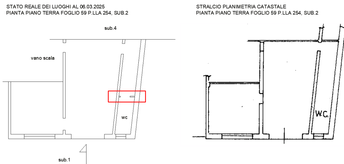
Figura 8 Confronto pianta piano terra sub. 2 Comune di Teggiano
