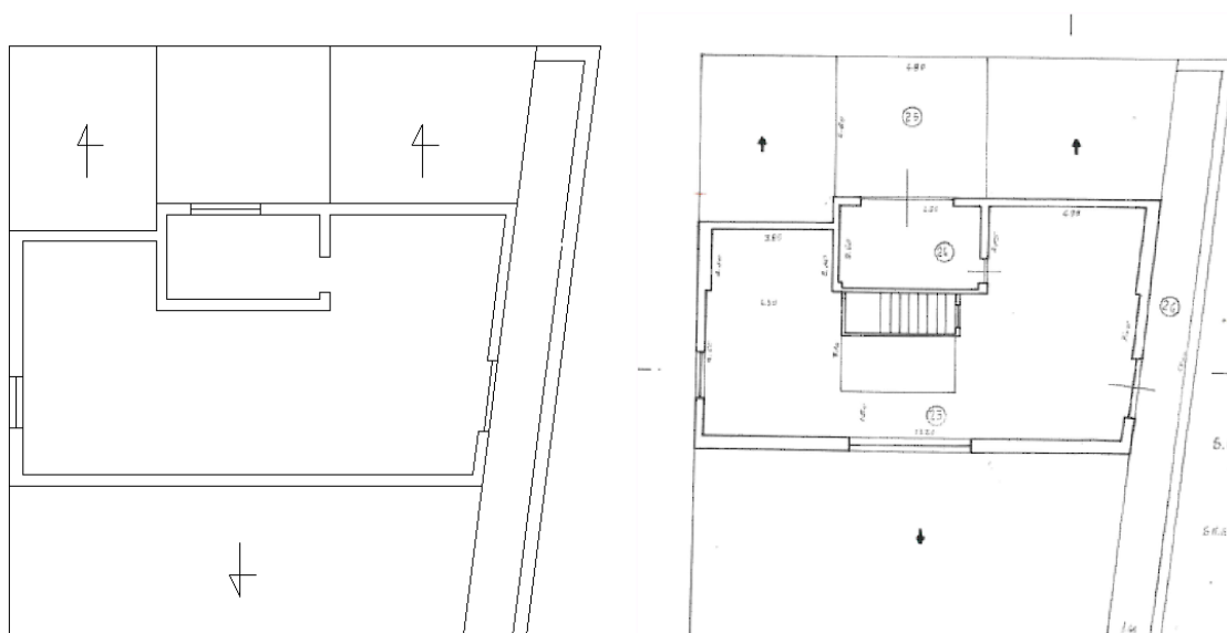
Figura 7 Confronto pianta piano secondo sub. 5 Comune di Teggiano
