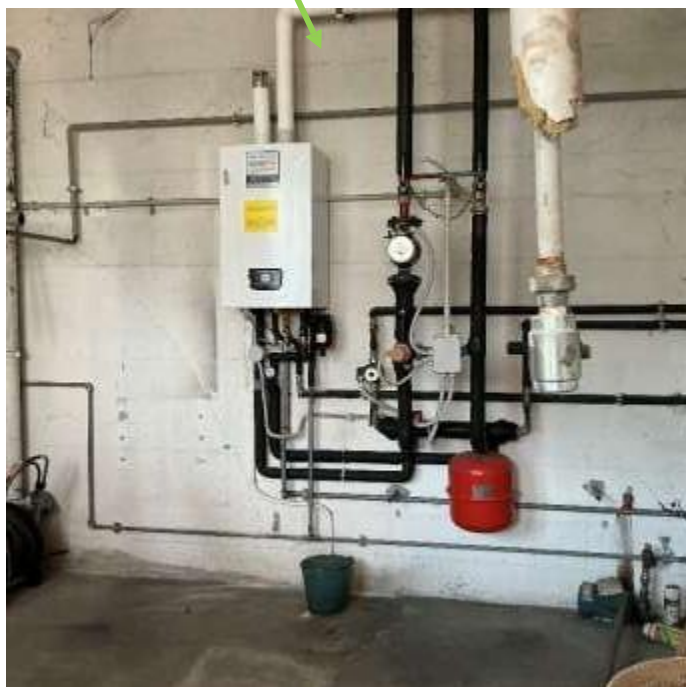
caldaia e impianti presenti all'interno del sub. 86, a servizio del sub. 87
