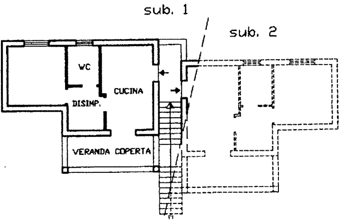
PIANO PRIMO h = 2,83
