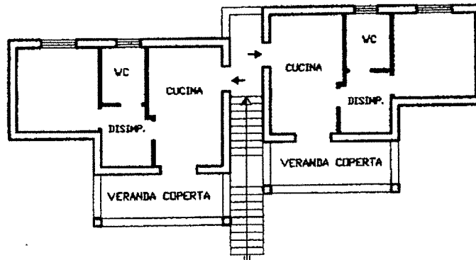
PIANO PRIMO h = 2,83
