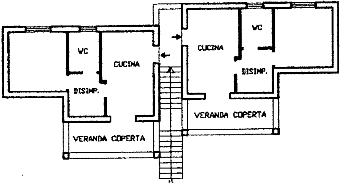
PIANO PRIMO h = 2,83
