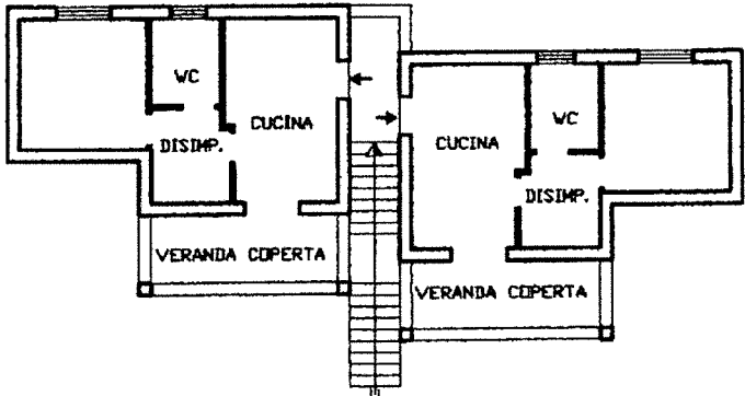
PIANO PRIMO h= 2,83
