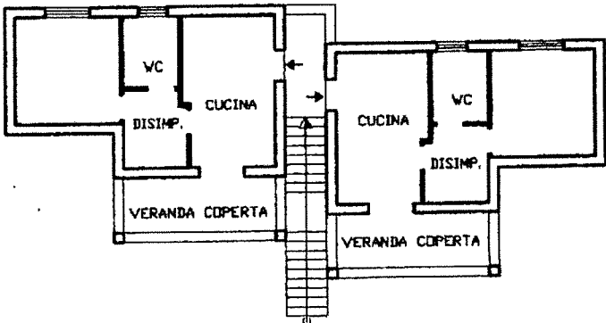
PIANO PRIMO h = 2,83
