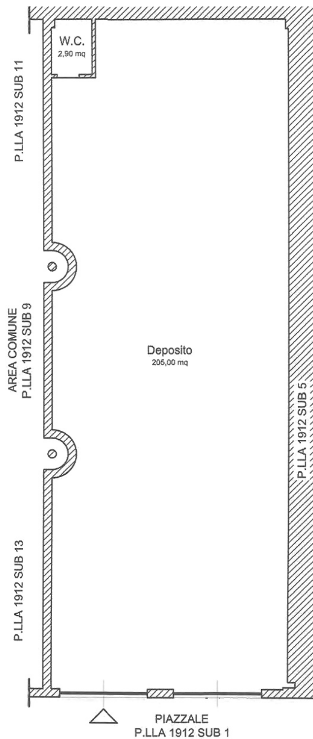
PIANTA DEPOSITO p.la 1912 sub 12
