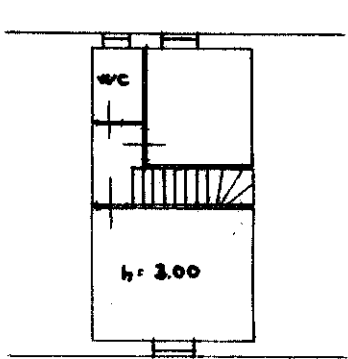
DIANO PRIMO
