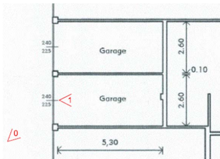
Planimetria autorimessa con indicazione dei punti di presa delle foto seguenti
