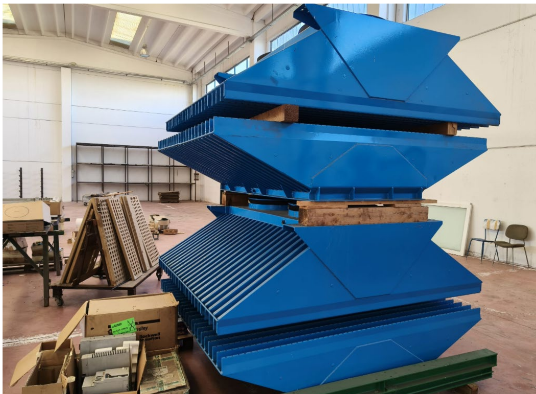
Foto 28 – Convogliatori aria
