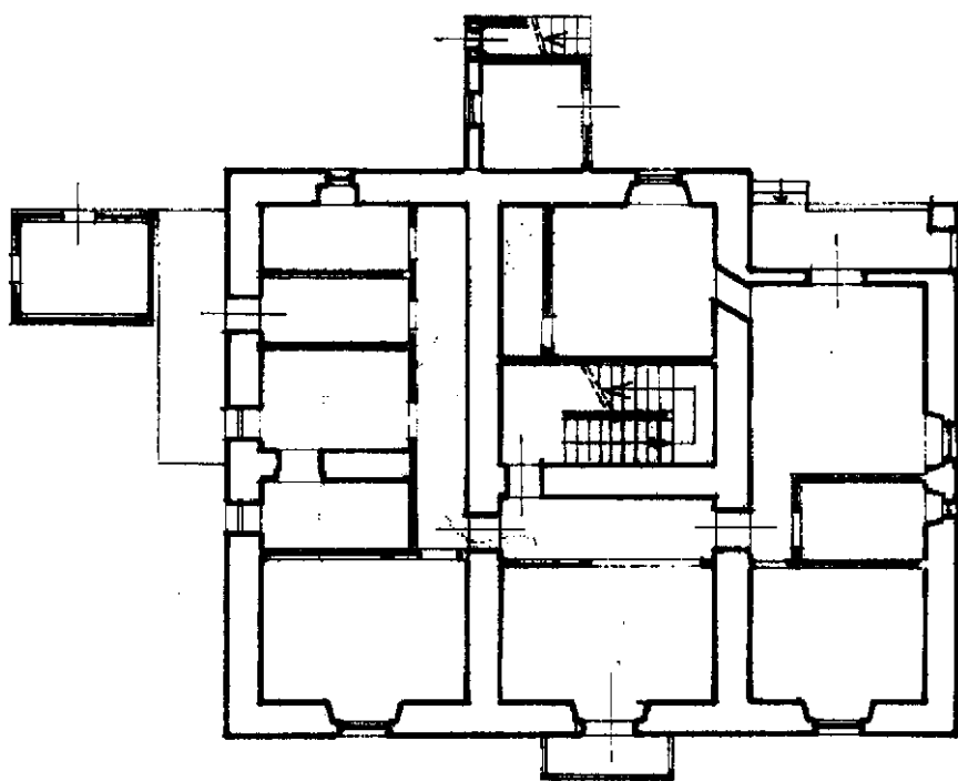
PIANTA PIANO PRIMO H=3,40
