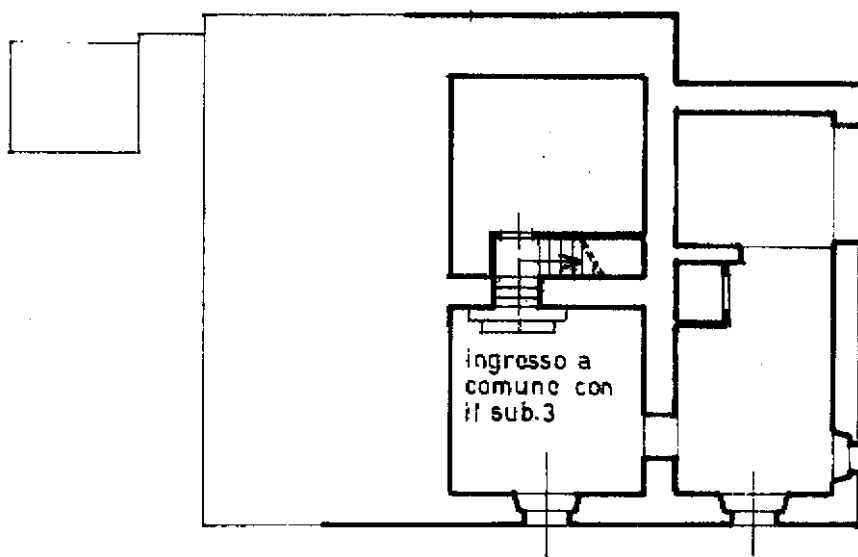
PIANTA PIANO TERRA H=3,50
