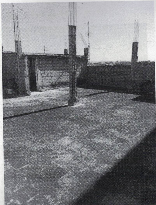
Foto 29- LASTRICO SOLARE VISTA OVEST - EST
