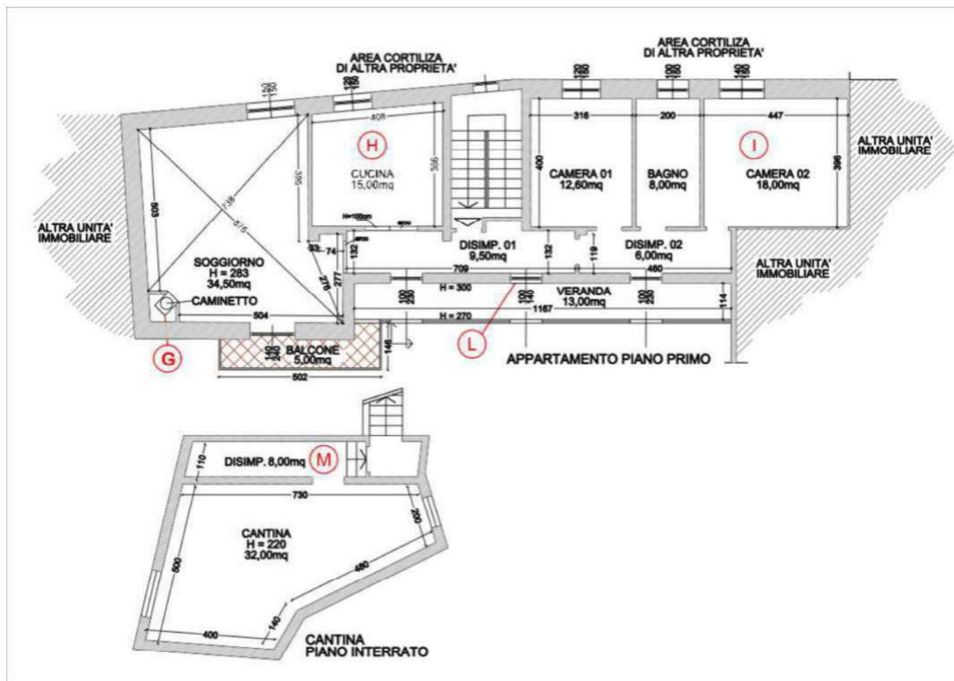
Pianta rilievo e difformità piano primo e cantina piano interrato.
