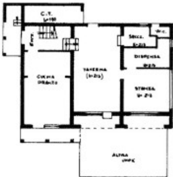
PIANTA PIANO TERRA - M. 280
