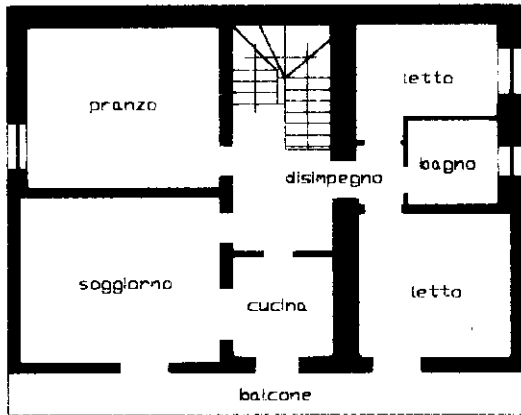
PIANTA PIANO PRIMO scala 1 : 200
