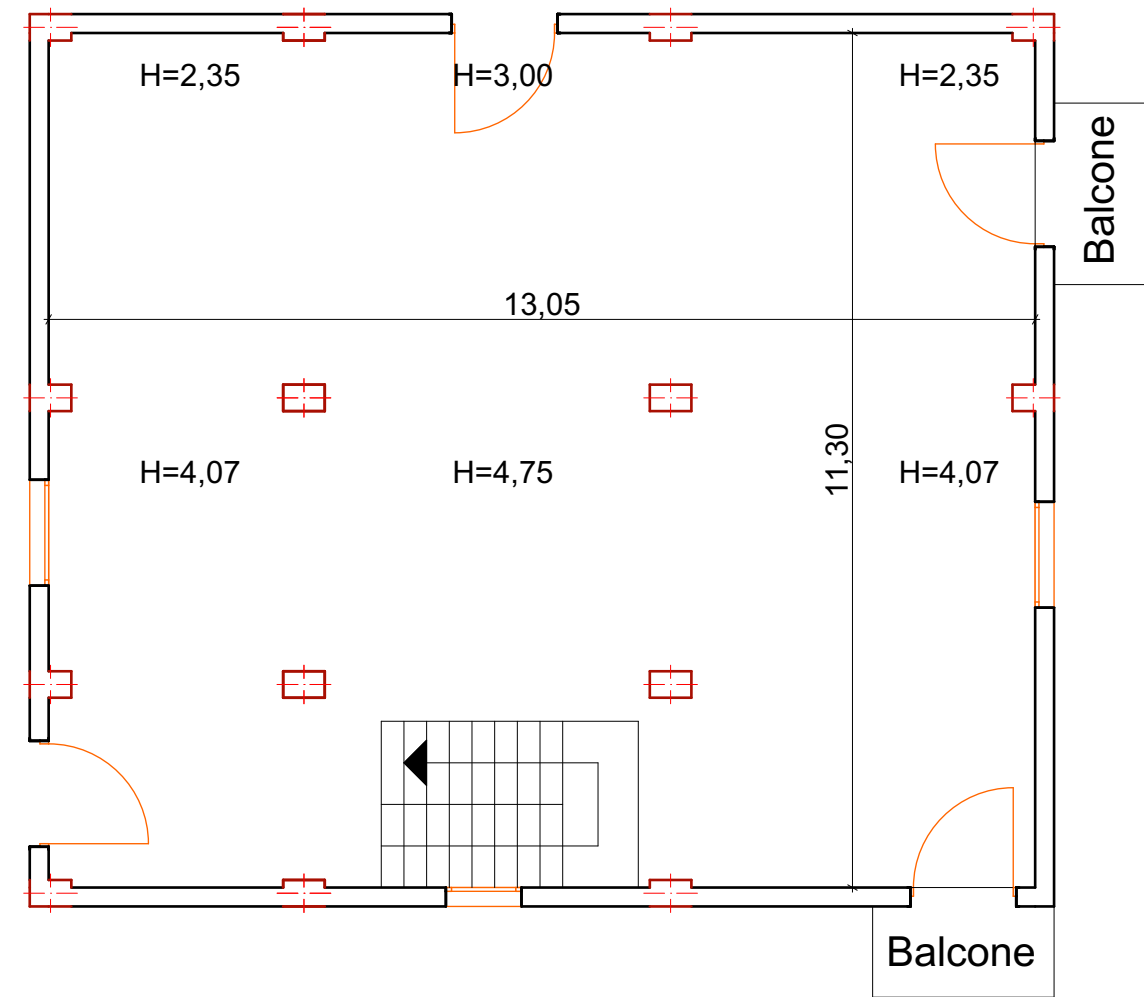
Piano Sototetto
