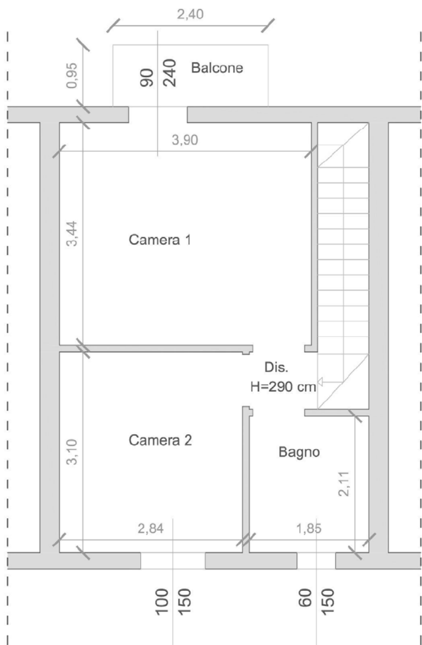
Fot. 2 – Pianta piano primo
