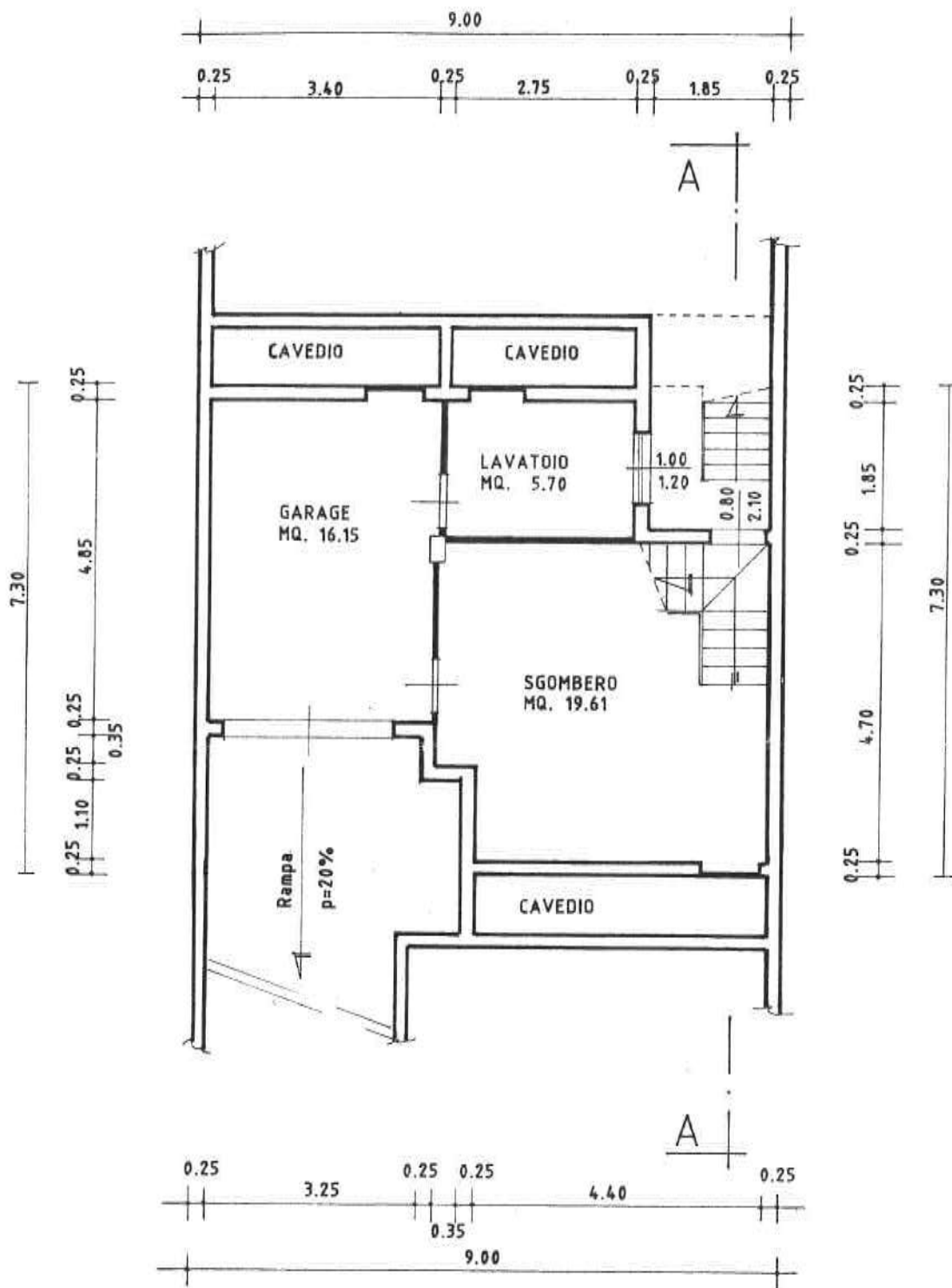
PIANTA PIANO CANTINA MODIFICATA
