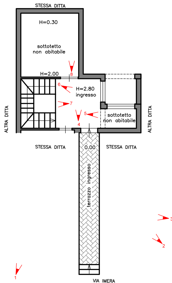
PIANTA PIANO TERRA via Imera p.a.e. PIANTA PIANO TERZO H=2.80
