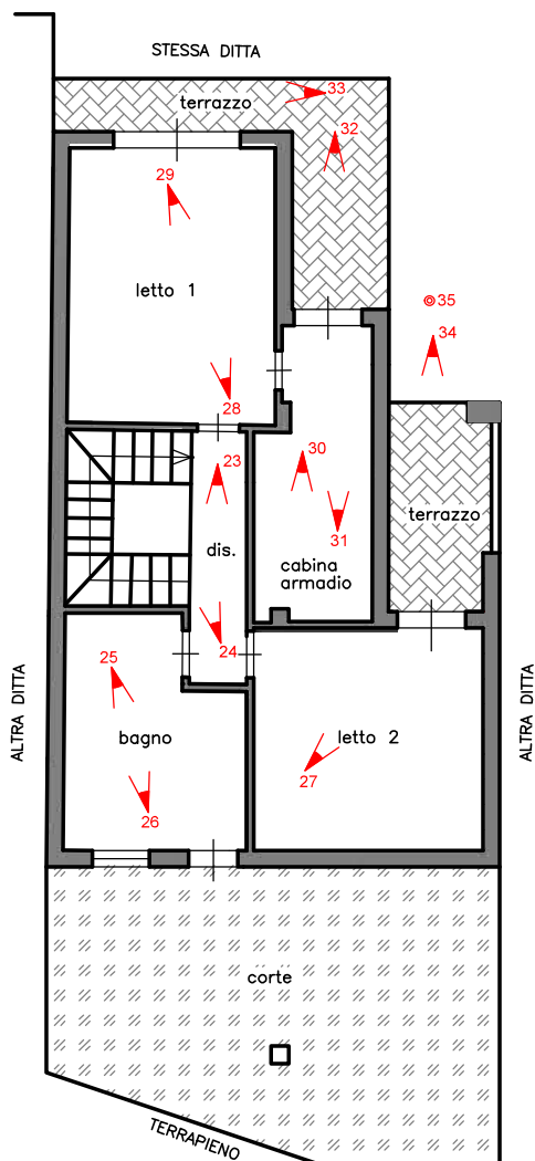
S.2.P. p.a.e. PIANTA PIANO PRIMO H=2.80
