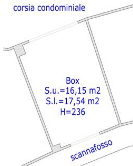
PIANTA STATO ATTUALE APPARTAMENTO PIANO INTERRATO
