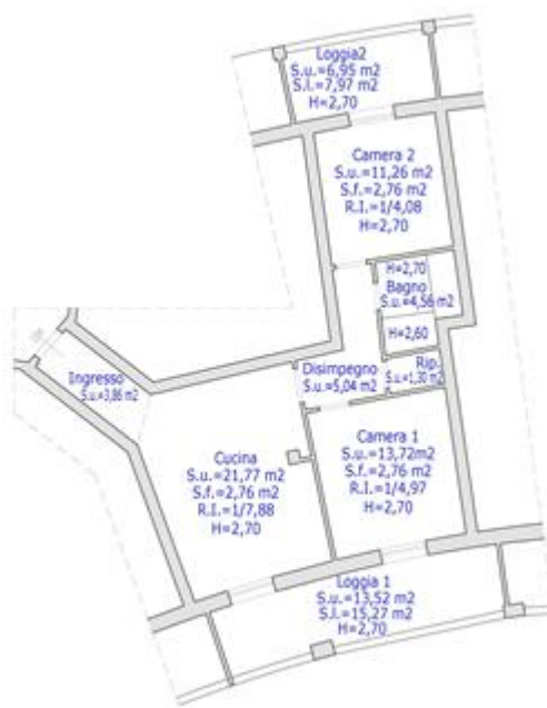
PIANTA STATO ATTUALE APPARTAMENTO PIANO PRIMO
