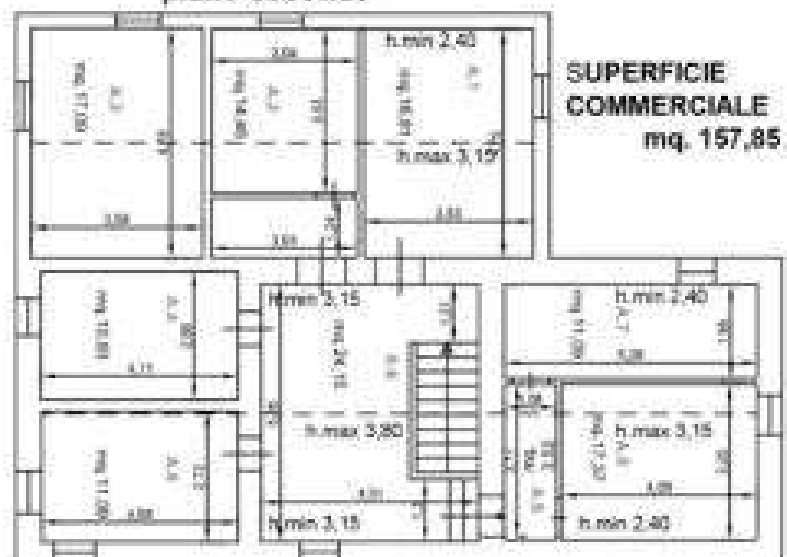
piano secondo
