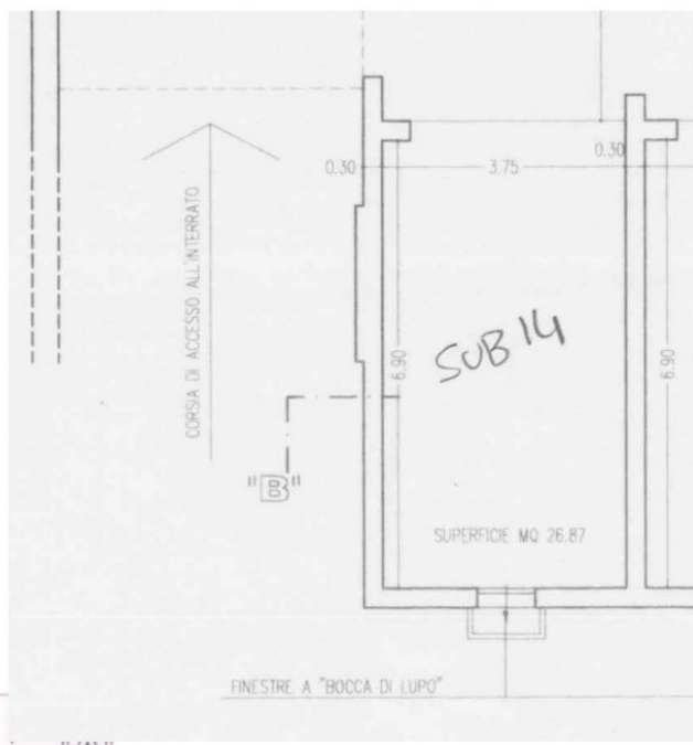
ESTRATTO PIANO INTERRATO
