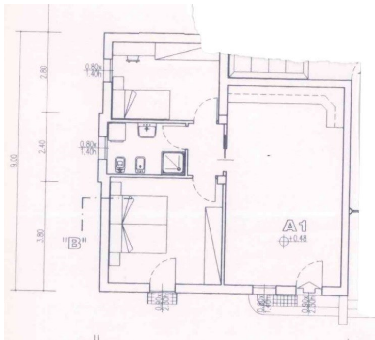
ESTRATTO PIANO TERRA
