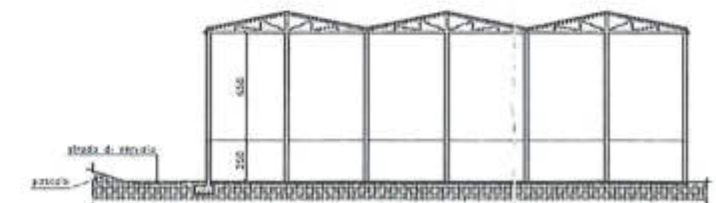
SEZIONE C-C'
