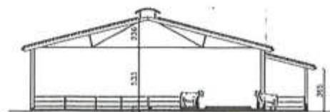
SEZIONE B-B'
