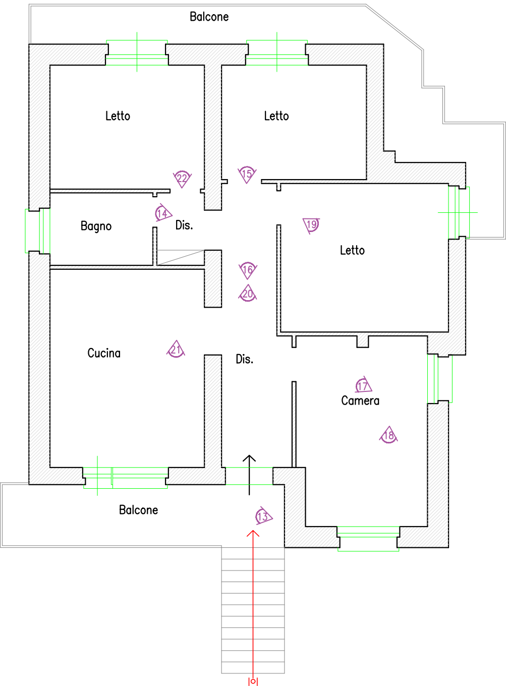
PIANTA 1:100 Piano Rialzato
