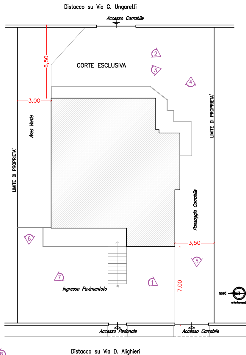
PLANIMETRIA GENERALE scala 1:200
