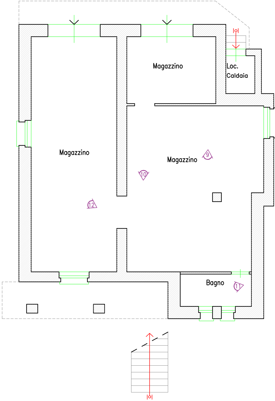
PIANTA 1:100 Piano Seminterrato
