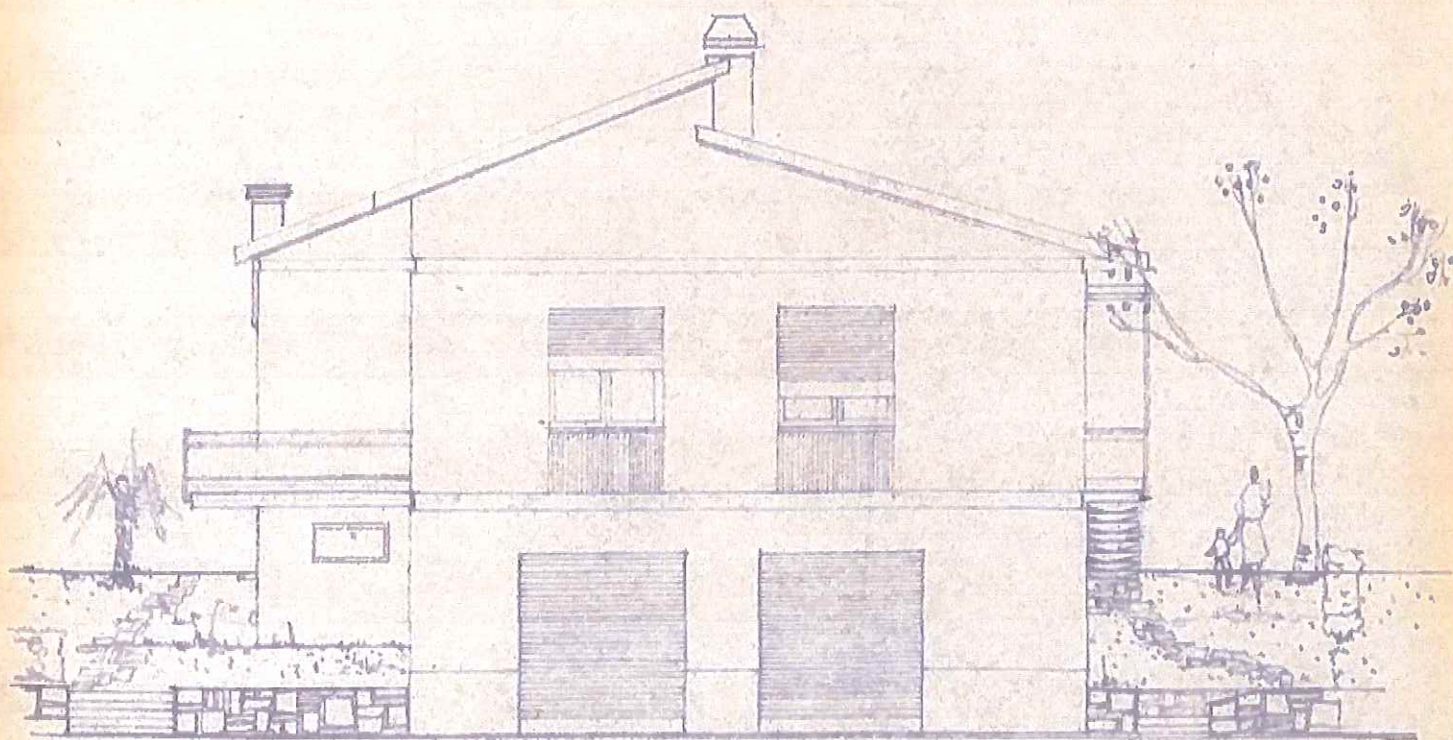
PROSPETTO N-E RAPP. 1/100
