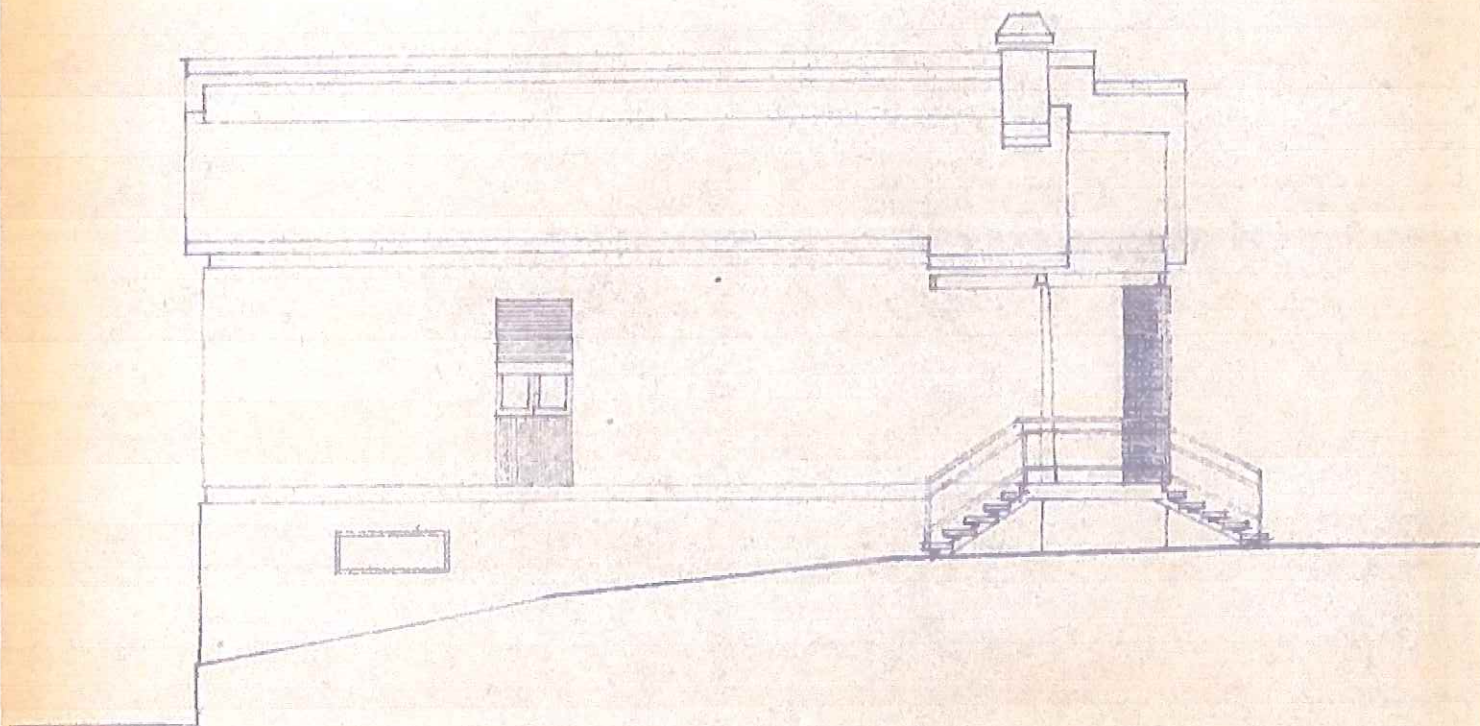
PROSPETTO N-O RAPP. 1/100
