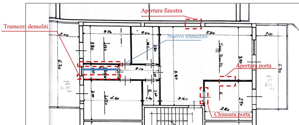
Pianta piano tipo – Concessione edilizia in Sanatoria n° 4 del 1998 ai sensi dell'aert. 13 L.47/85
