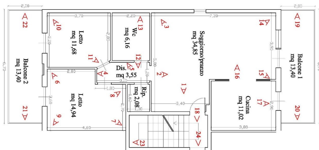
Pianta piano secondo - Rilievo effettuato dal sottoscritto CTU
