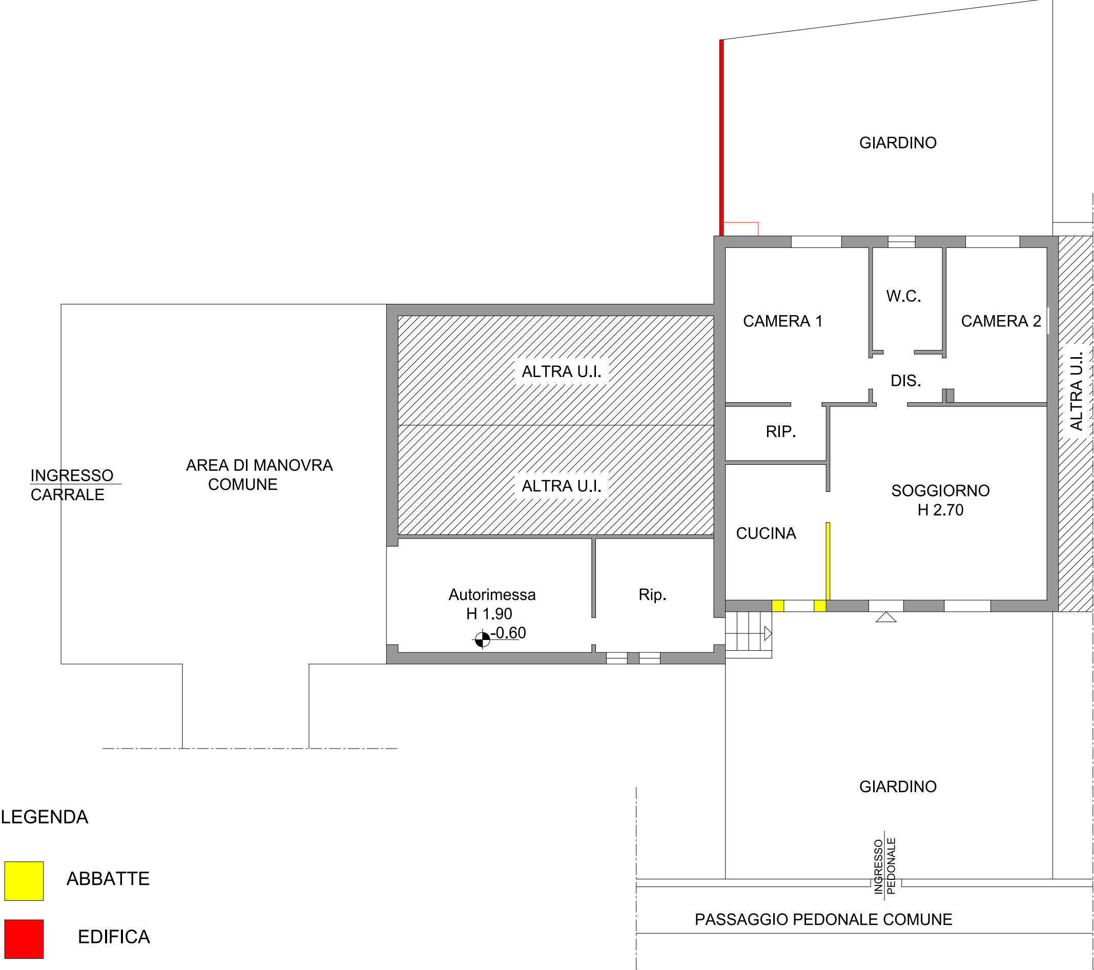
PIANTA PIANO TERRA (COMPARAZIONE TRA STATO DI FATTO E C.E. 281/1 DEL 05/05/84)
