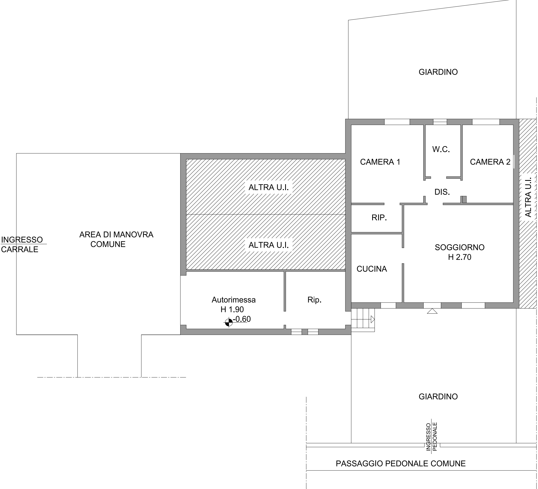
PIANTA PIANO TERRA COME DA C.E. N. 282/1 DEL 05/05/84
