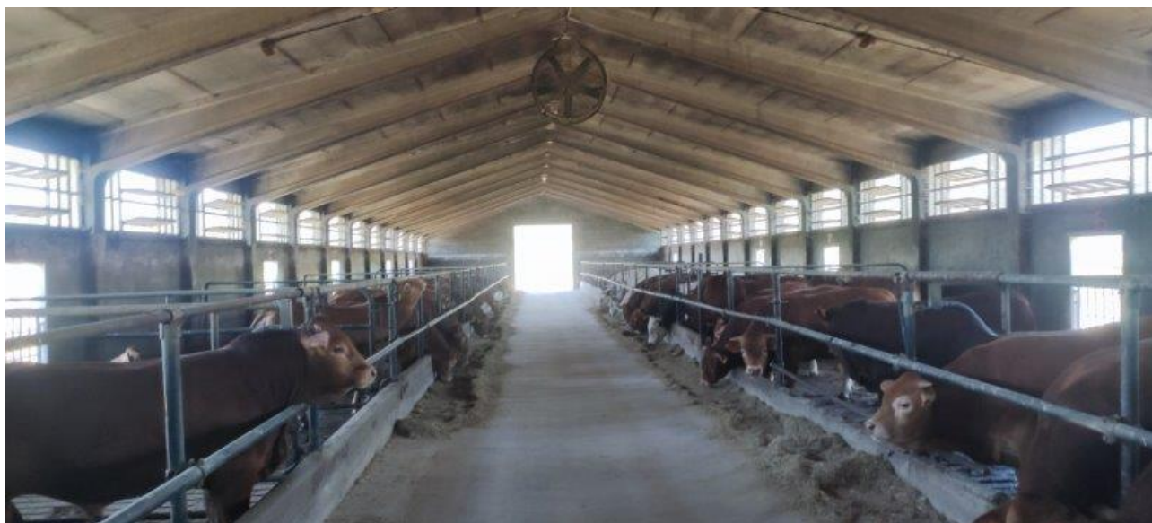
Figura 3 CORSIA ALIMENTAZIONE STALLA PER BOVINI
