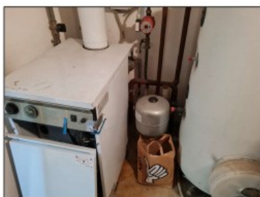
FOTO 98 - CALDAIA TRADIZIONALE MARCA RIELLO
