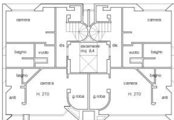
PIANO SECONDO
