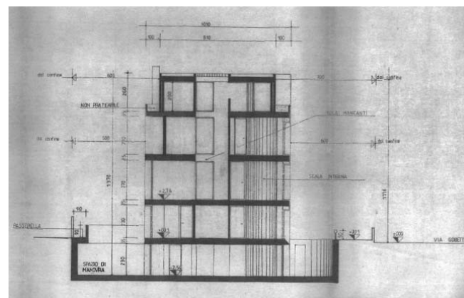
SEZIONE BB (variante a C.E. N°220/1989)
