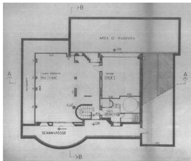
PIANO INTERRATO (variante a C.E. N°220/1989)
