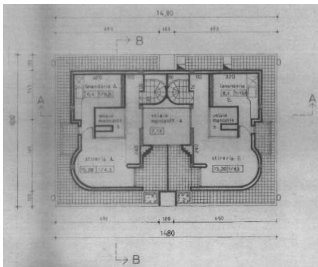
PIANO TERZO SOTTOTETTO
