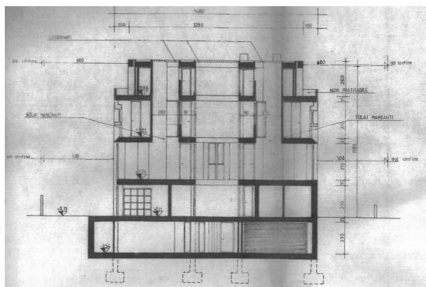
SEZIONE AA
