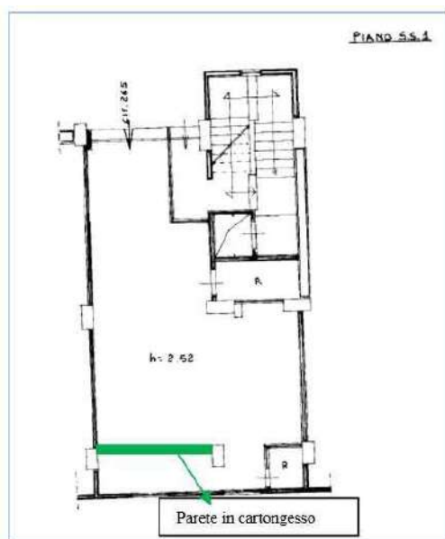
Planimetria Catastale Garage con indicate le difformità
