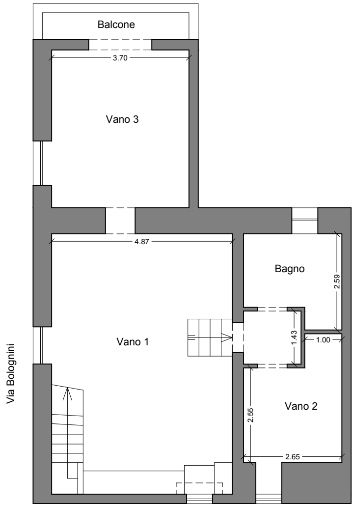
PIANTA PIANO PRIMO - STATO DI FATTO RAPP. 1:100
