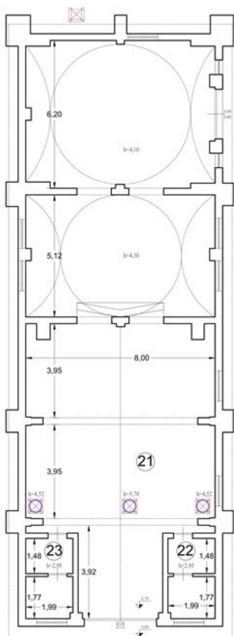
Stato di fatto
