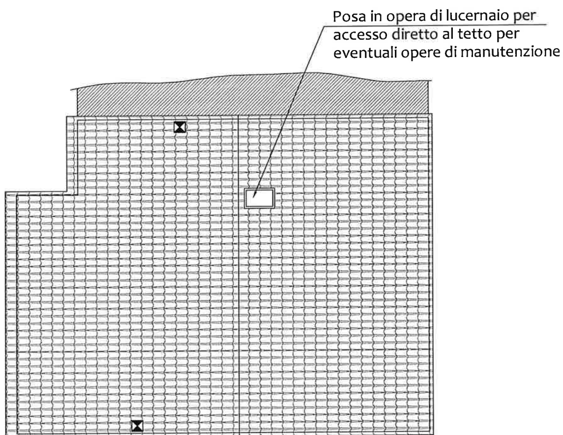
PIANTA COPERTURA
