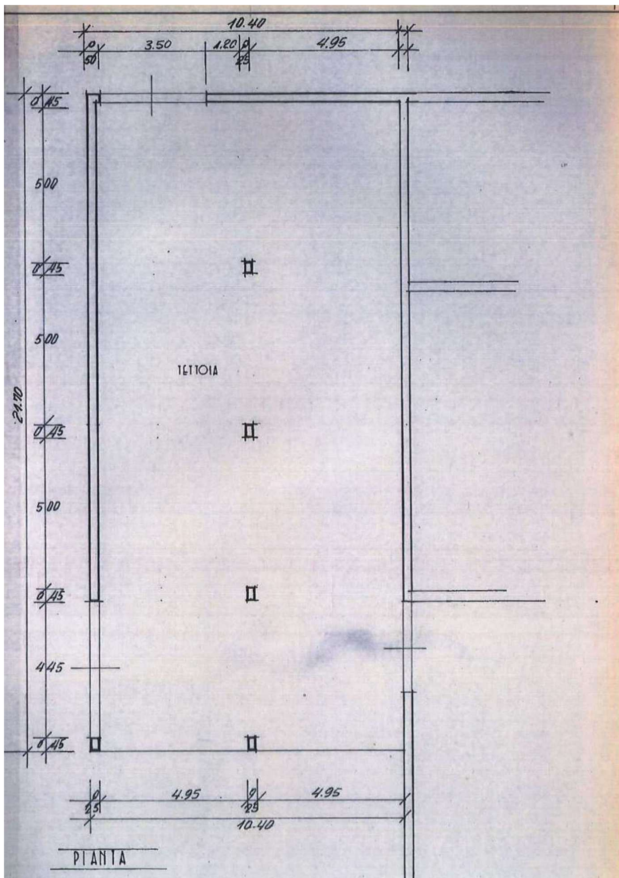
Planimetria del progetto del corpo di fabbrica a lato ovest, in larga parte crollato, mappale 218, subalterno 6, del foglio 24.
