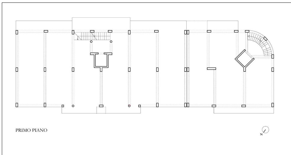
Fig. 13 - Piano primo. Rilievo dello stato di fatto.
