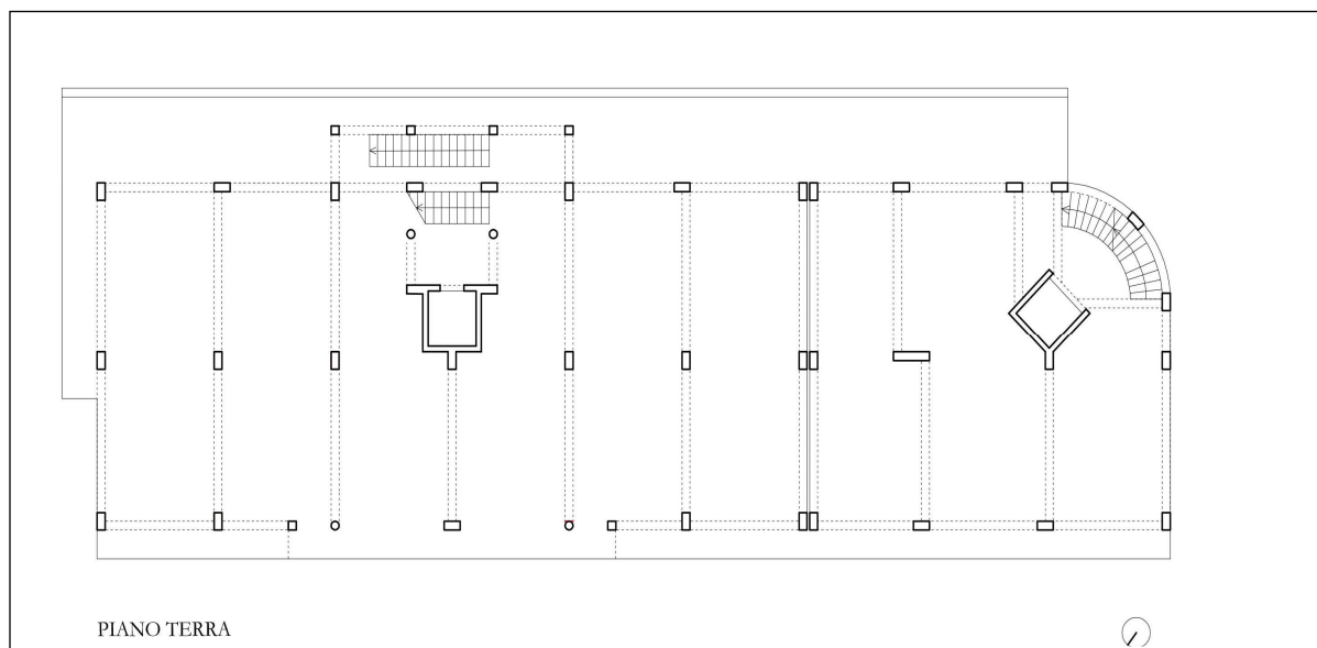
Fig. 10 - Piano Terra. Rilievo dello stato di fatto.
