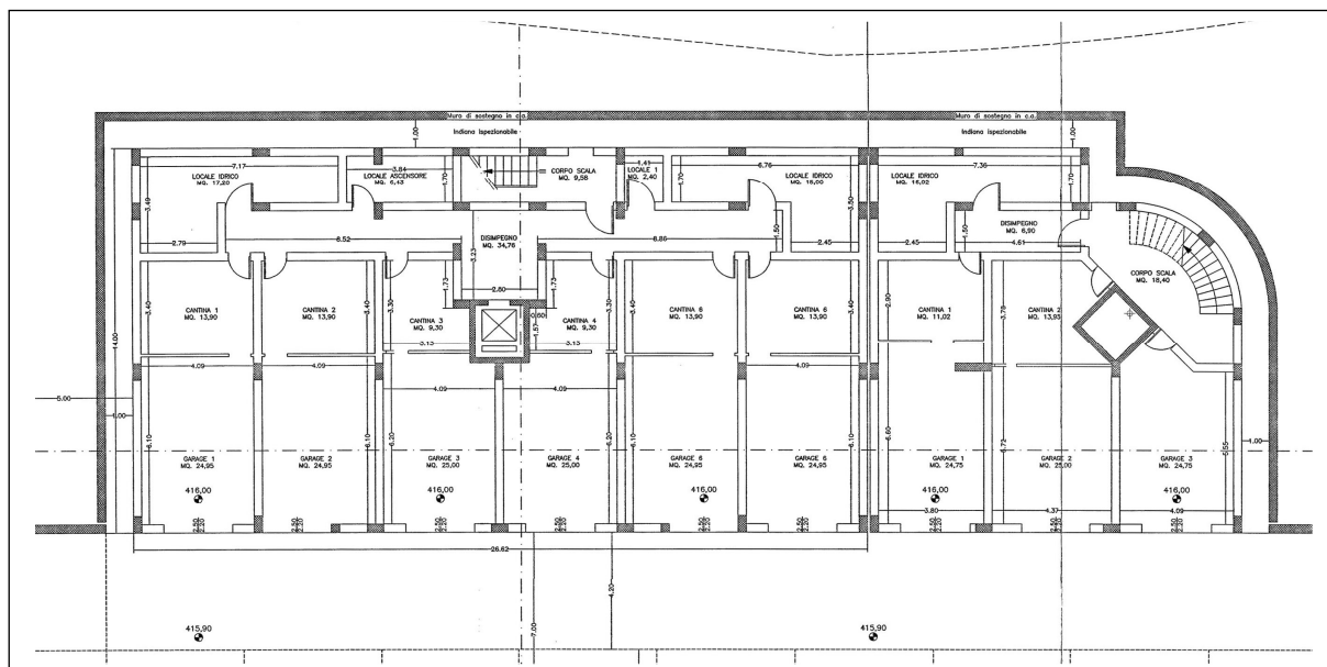
Fig. 9 - Piano S1 seminterrato. Variante del 2010
