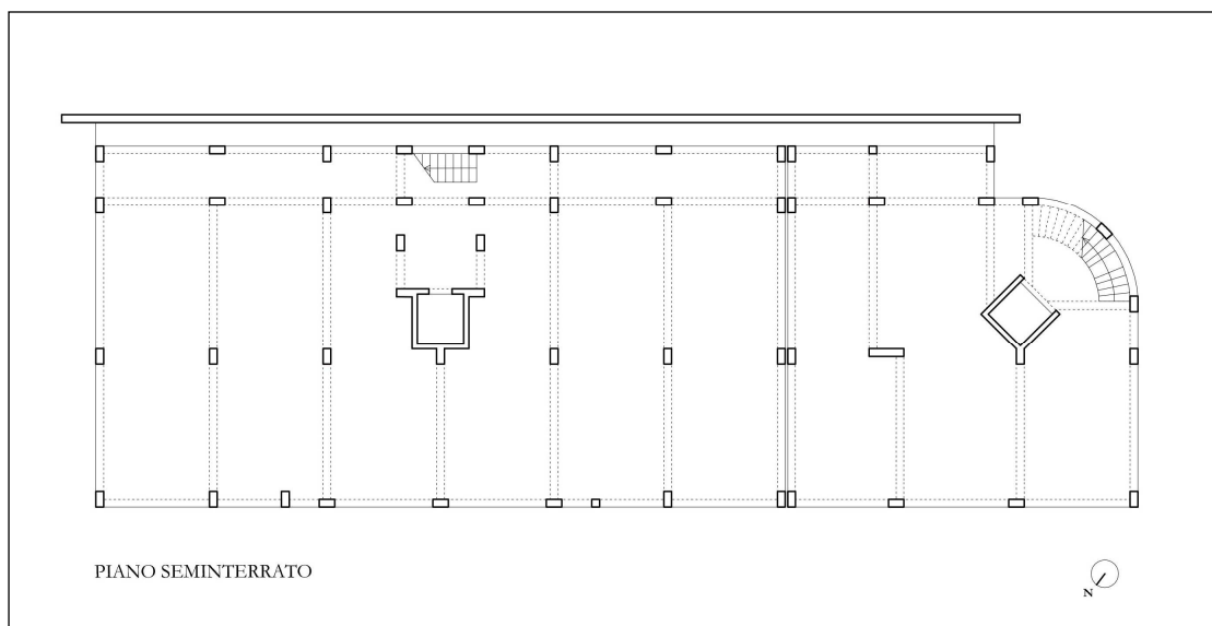
Fig. 3. Fabbricato pignorato in corso di costruzione. Rilievo dello stato di fatto. Piano seminterrato S1
