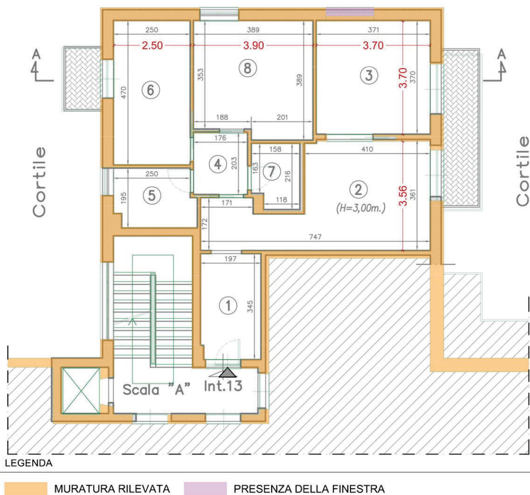
gr.5.02: sovrapposizione pianta C.I.L.A prot.25933 e pianta stato di fatto
