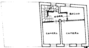
PIANTA PIANO PRIMO H=2.55
