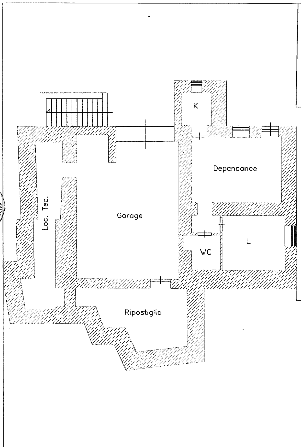
Planimetria di rilievo garage e depandance
